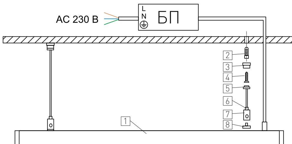
Рис. 2. Установка и подключение светильника
