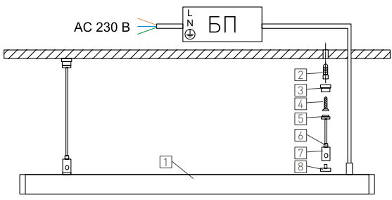
Рис. 2. Монтаж светильника
