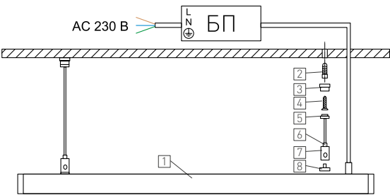
Рис. 2. Монтаж светильника
